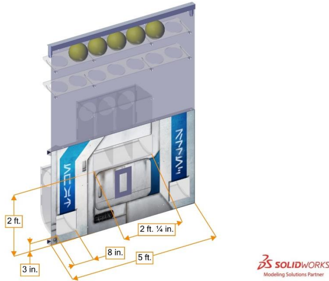
Şekil 3-13 YÜKLEME BÖLMESİ
