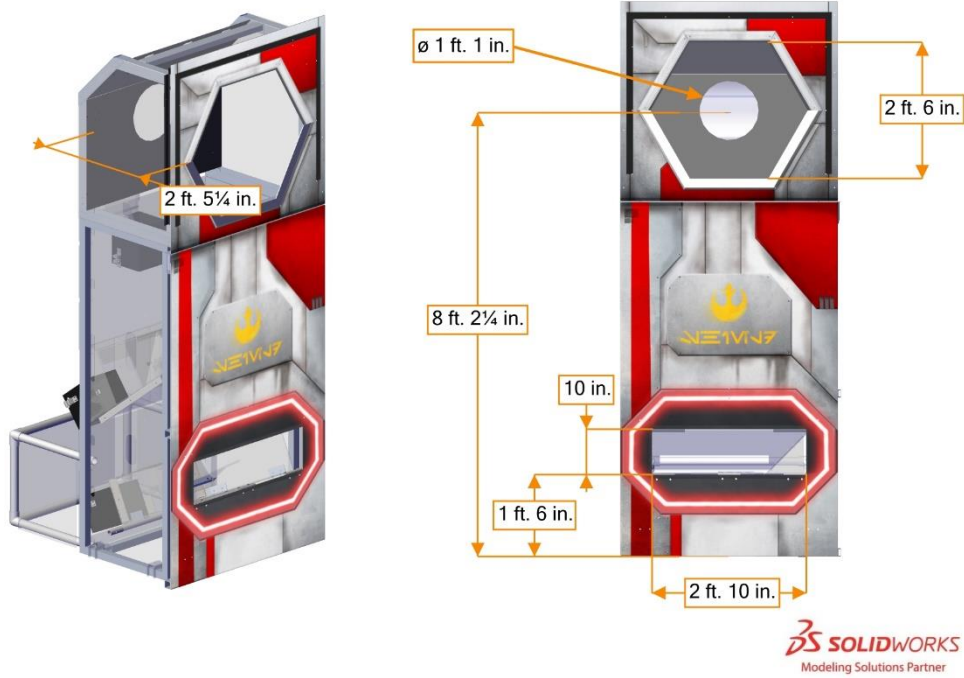
Şekil 3-15 GÜÇ GİRİŞİ boyutları
