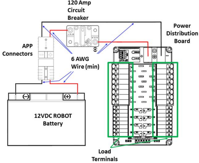
Şekil 9-10 Elektrik bağlantı şeması
