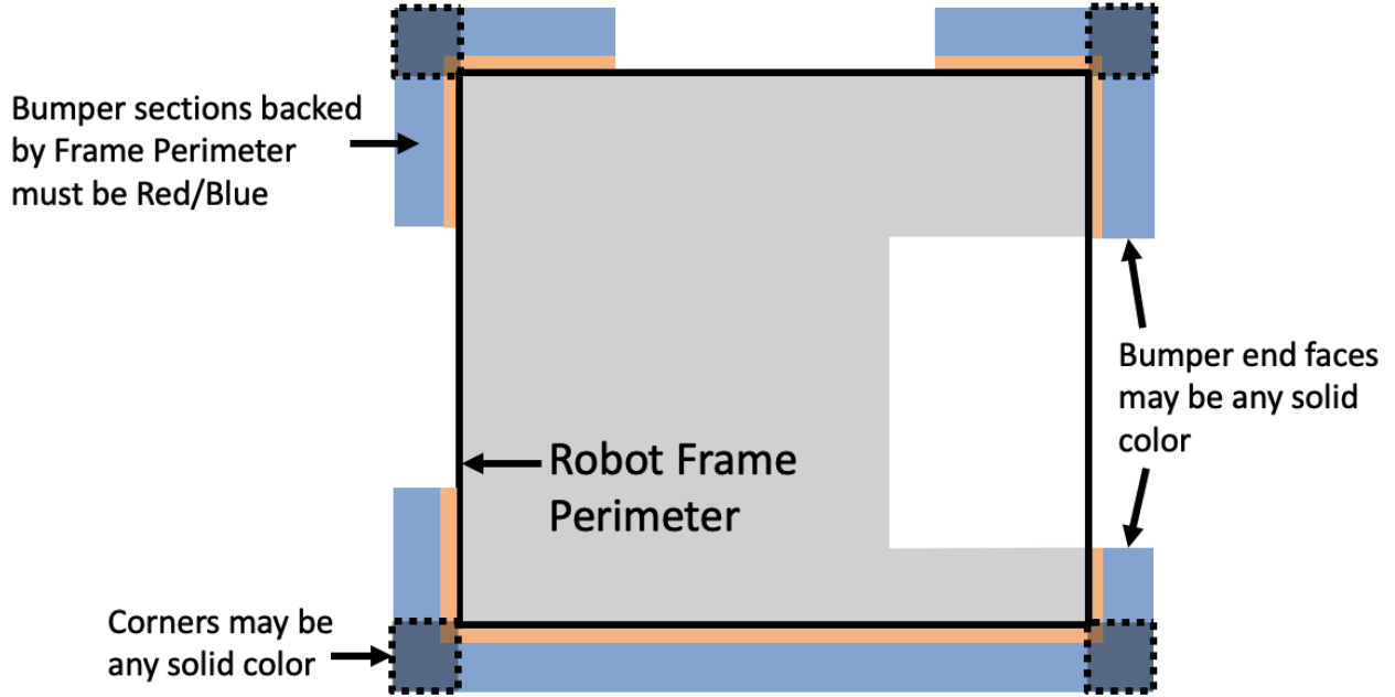
Şekil 9-4 TAMPON renk örneği
