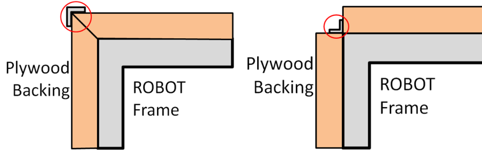
Şekil 9-6 TAMPON uçlarındaki sert parçalar
