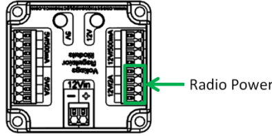
Şekil 9-12 Radyo güç kaynağı
