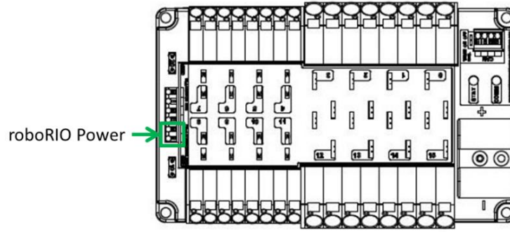
Şekil 9-11 roboRIO güç kaynağı
