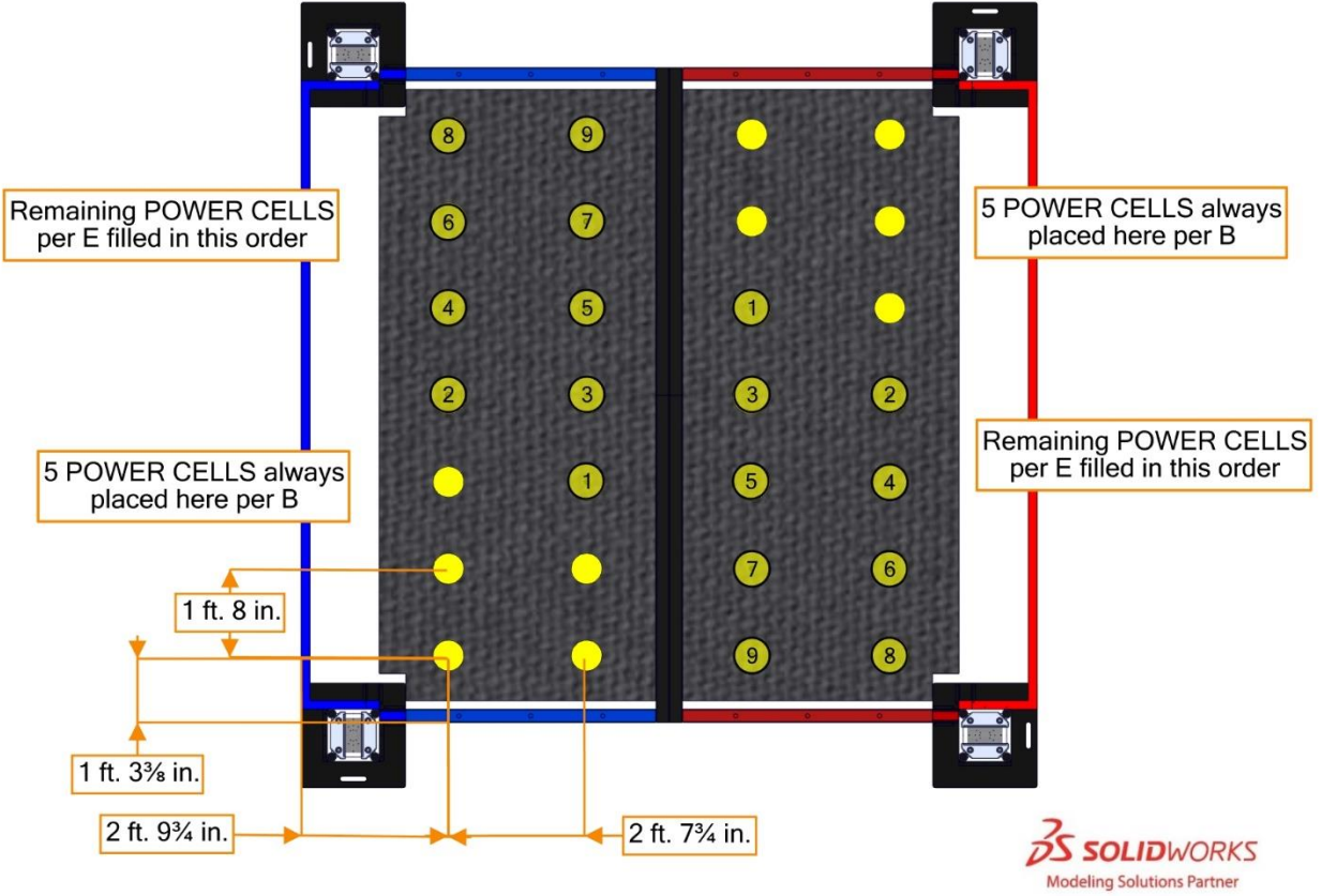
Şekil 4-2 RANDEVU NOKTASındaki GÜÇ HÜCRESİ yerleşimi
