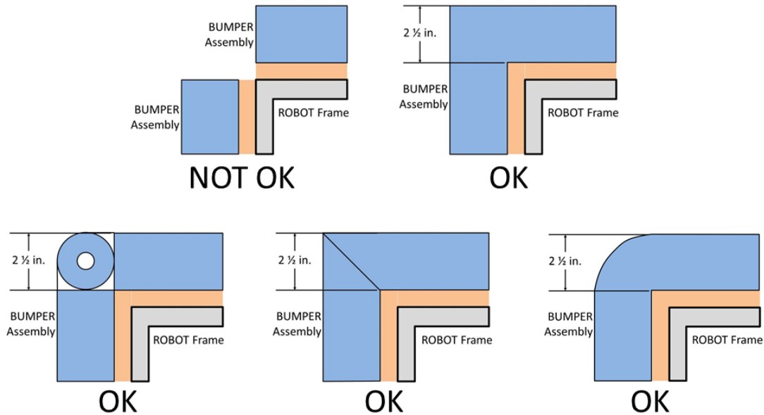
Şekil 9-8 TAMPON köşelerindeki yumuşak parçalar
