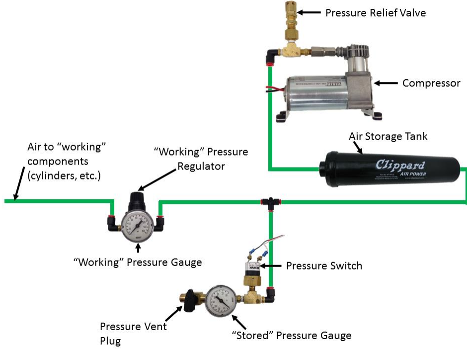
Şekil 9-15 Pnömatik devre örneği
