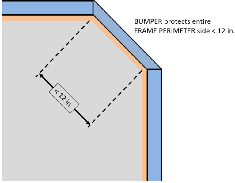
Şekil 9-3 Tüm kenarları/köşeleri içeren TAMPON
