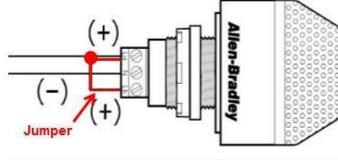
Şekil 9-14 RSL kablo bağlantısı
