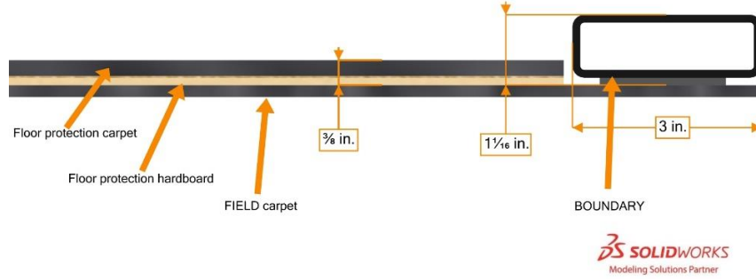
Şekil 3-11 Zemin koruması düşey kesit
