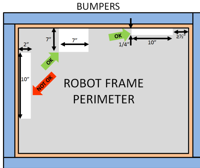
Şekil 9-9 TAMPON destek örnekleri
