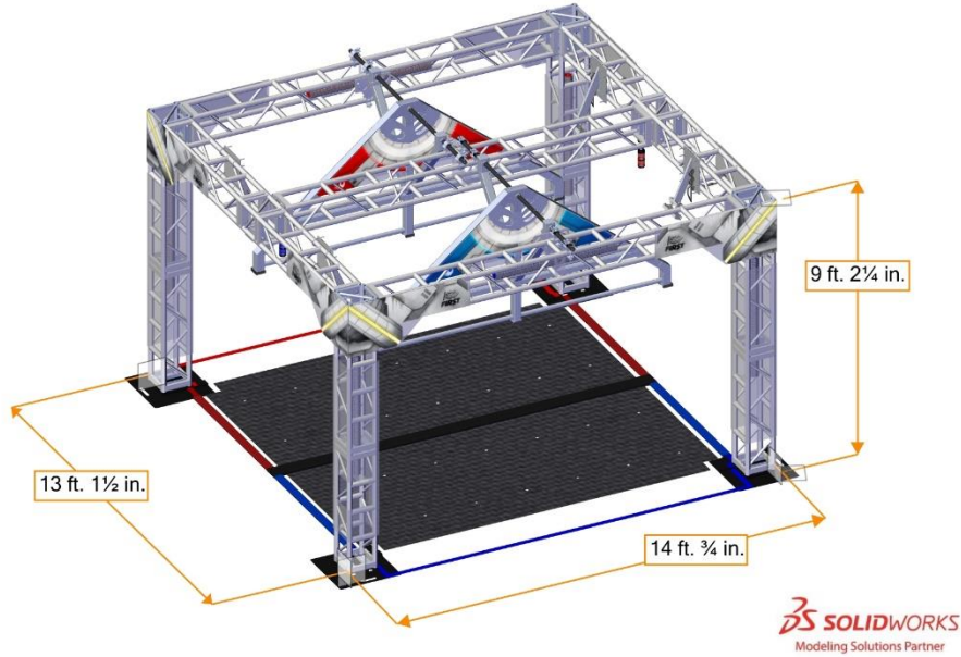
Şekil 3-7 KALKAN JENERATÖRÜ yapısı
